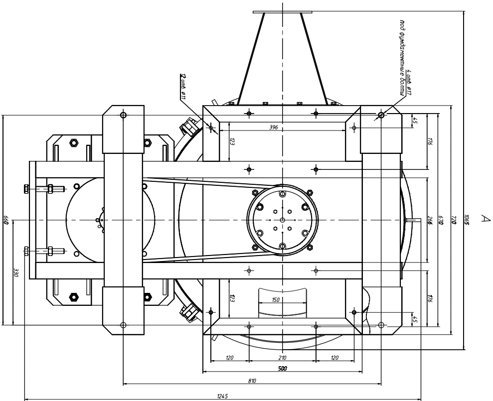
Рис. 2 (1:10) Схема стиральной мельницы с двигателем
