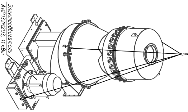
Рис. 1 (1:10) Схема стиральной мельницы
